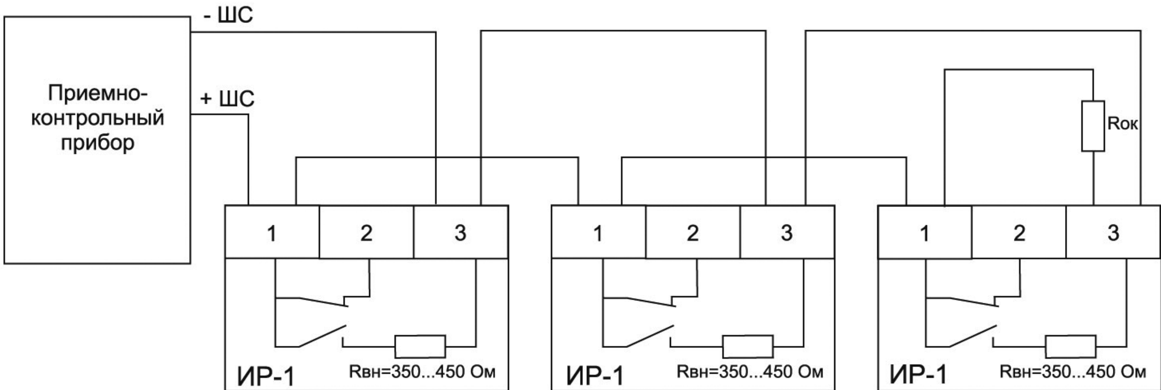
Схема включения извещателя ИР-1 в приемно-контрольный прибор со постоянными ШС по схеме индикации без "квитирования"
