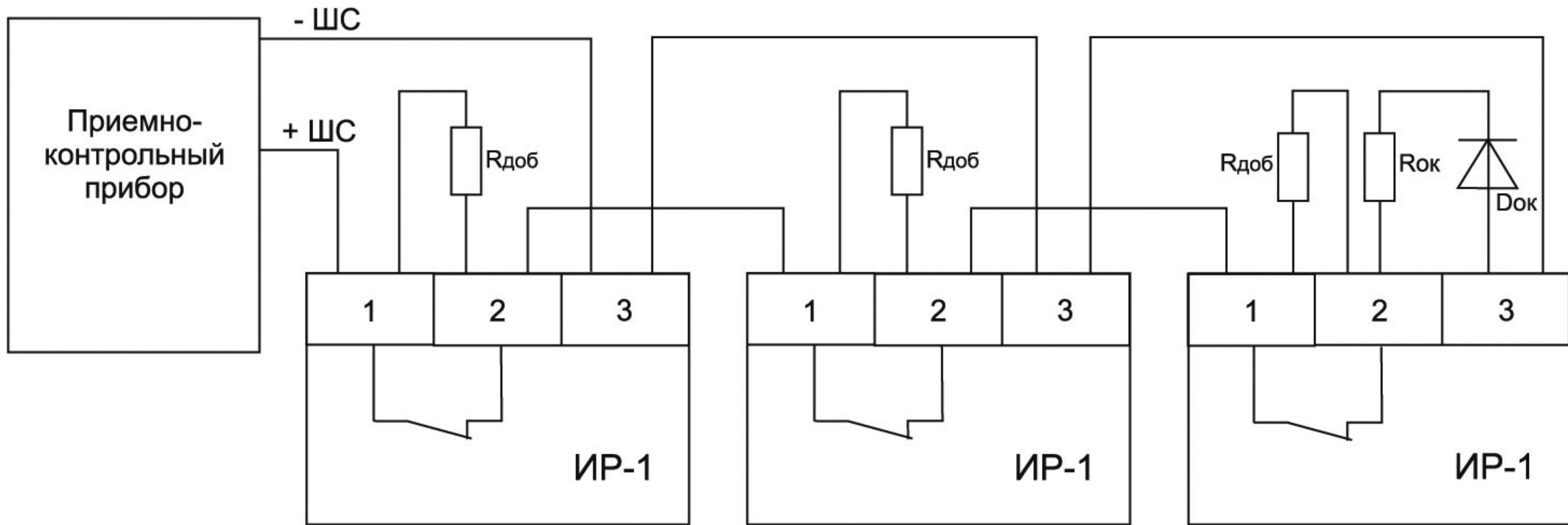
Схема включения извещателя ИР-1 в приемно-контрольный прибор со знакопеременными ШС по схеме индикации с "квитированием"
