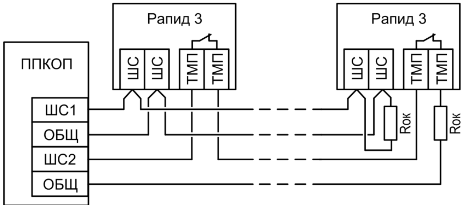
Схема подключения извещателей к ППКОП
