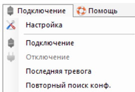
РИС. 9 Меню «Подключение»
