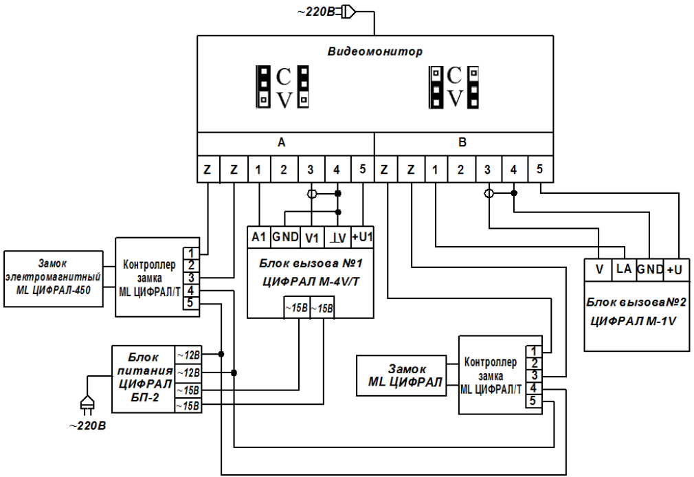
Рисунок А.3. Подключение видеомониторов ЦИФРАЛ VM-3020, ЦИФРАЛ VM-3021 к блоку вызова с видеоканалом.
