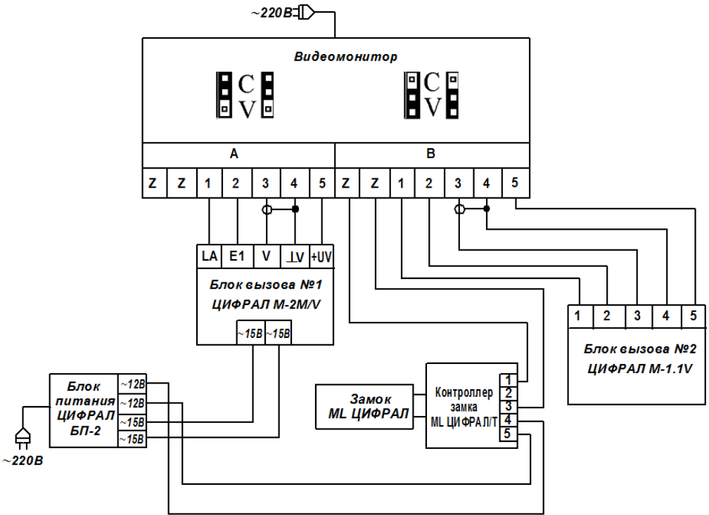
Рисунок А.1. Подключение видеомониторов ЦИФРАЛ ВМ-3020, ЦИФРАЛ ВМ-3021 к блоку вызова прямой адресации и к блокам вызова с видеоканалом.
