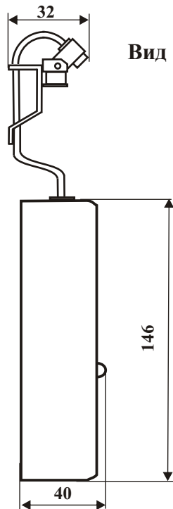
Рис 4 Извещатель пожарный пламени “Пульсар 1-011Н”, “Пульсар 1-011С” со снятой розеткой
